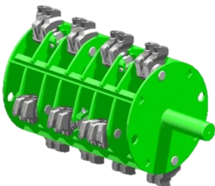
Rotor équipé de 28 fléaux forestiers mobiles
