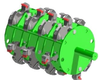
Rotor équipé de 14 outils coupants fixes
