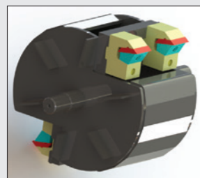
Broyage par rotor équipé de 3 couteaux fixes de 50 mm et 1 contre-lame réglable
